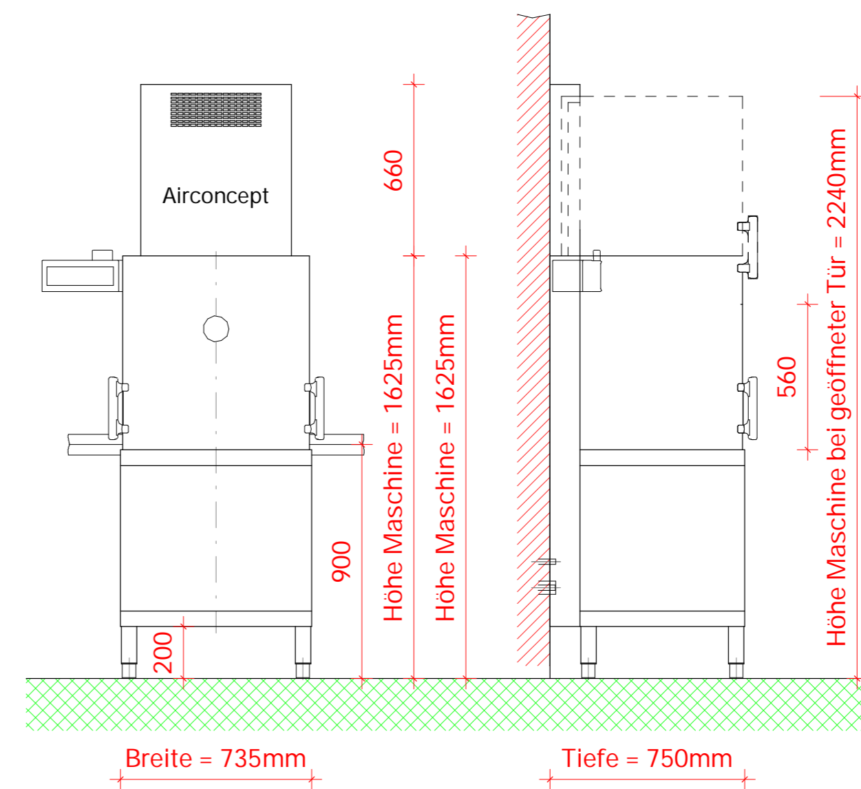
Detailschema Spülmaschine Massstab 1:20
